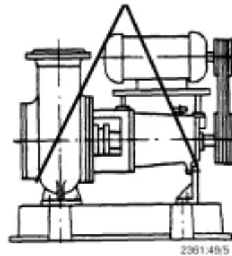
Рис. 3.1-3 Транспортировка насосного агрегата в сборе
